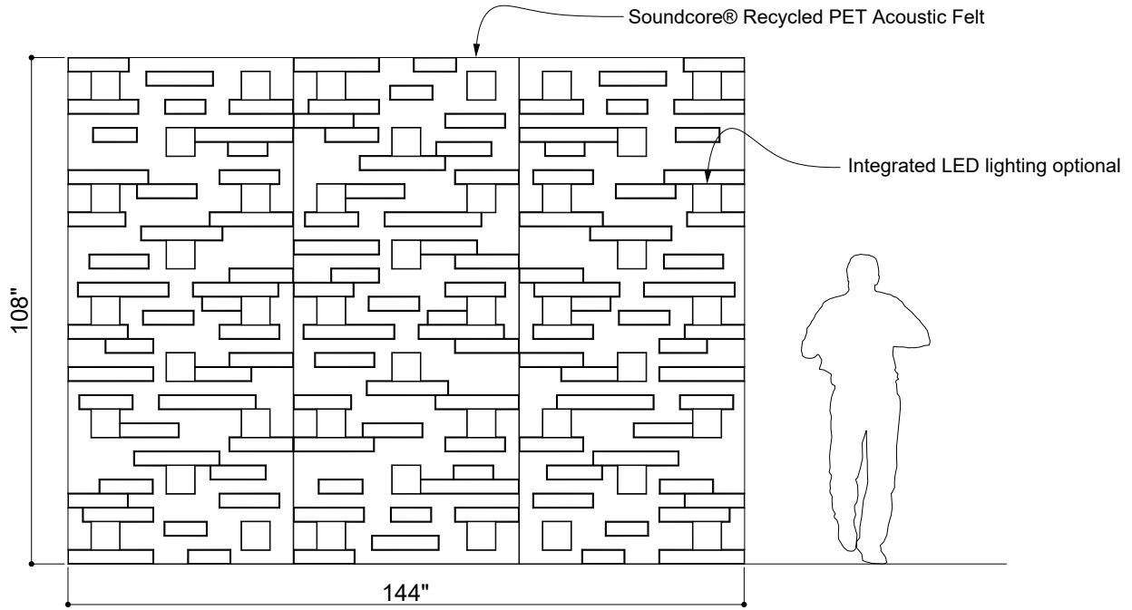
① ELEVATION 1
