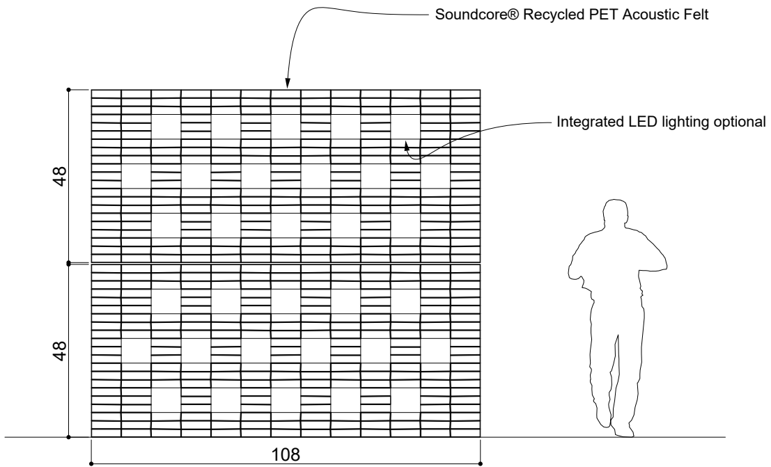
② ELEVATION 2
